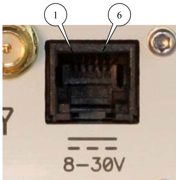
Рис.2.6.2 Разъём RJ11
