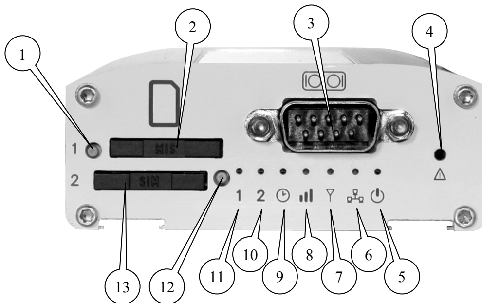
Рис.2.5.1 Вид спереди.
