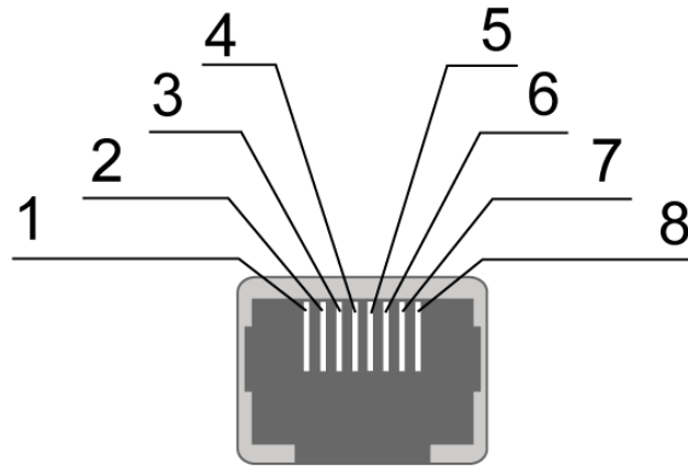
Рис. 3.7. Ethernet-разъём
