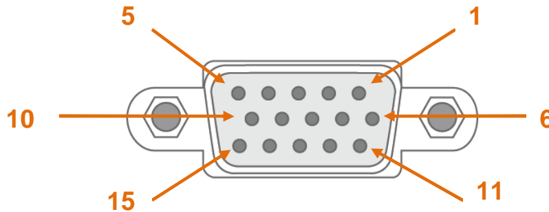
Рис. 2.5.1. Разъём DB15
