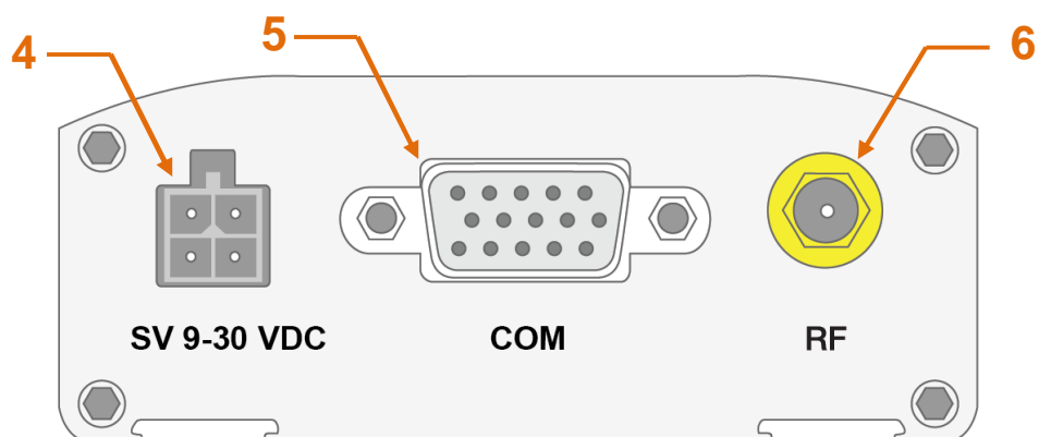
Рис. 2.4.2. Вид сзади
