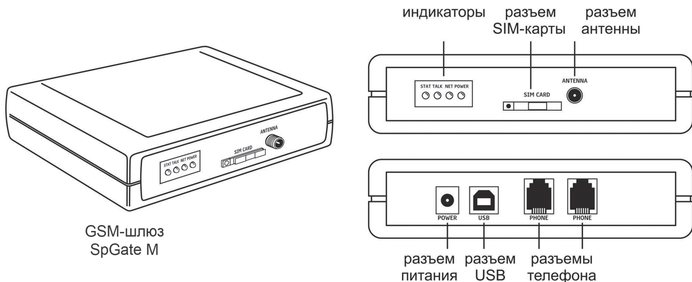
Рисунок 2.1. GSM-шлюз SpGate M
