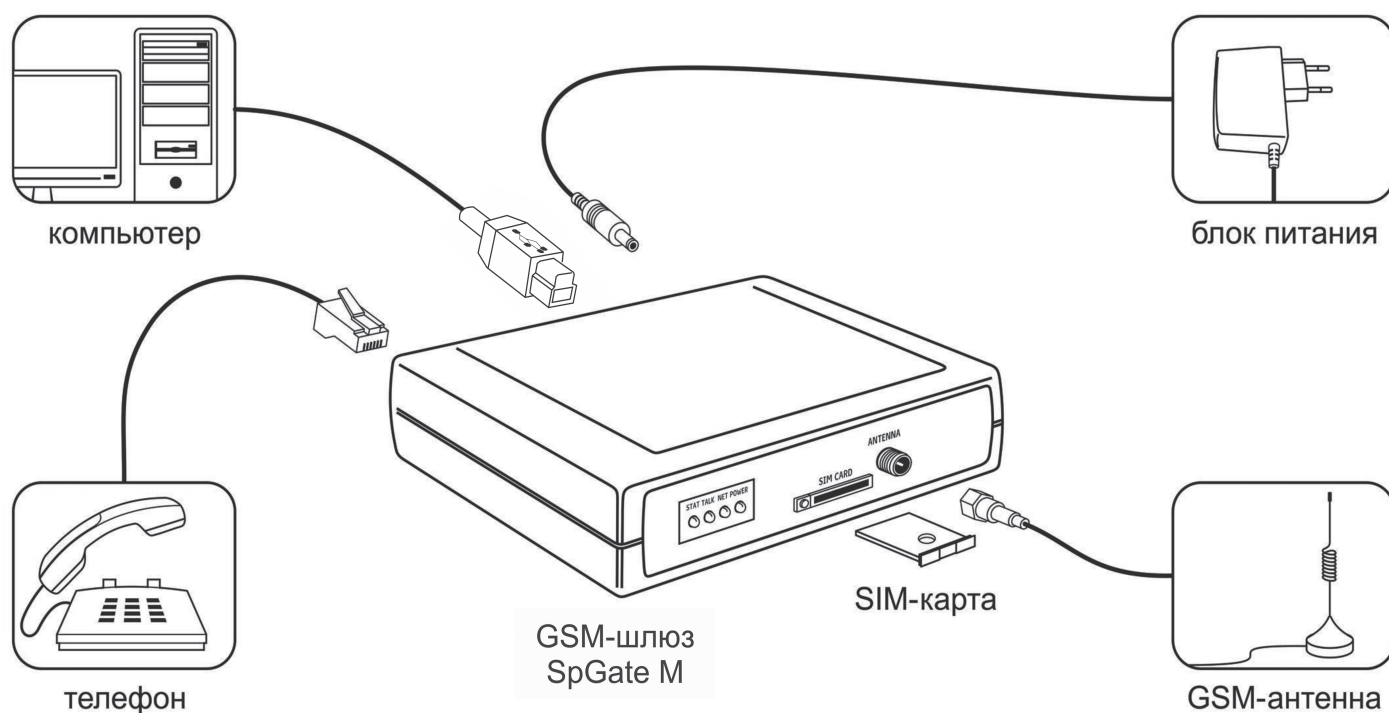
Рис 6.1 Подключение шлюза SpGate M
