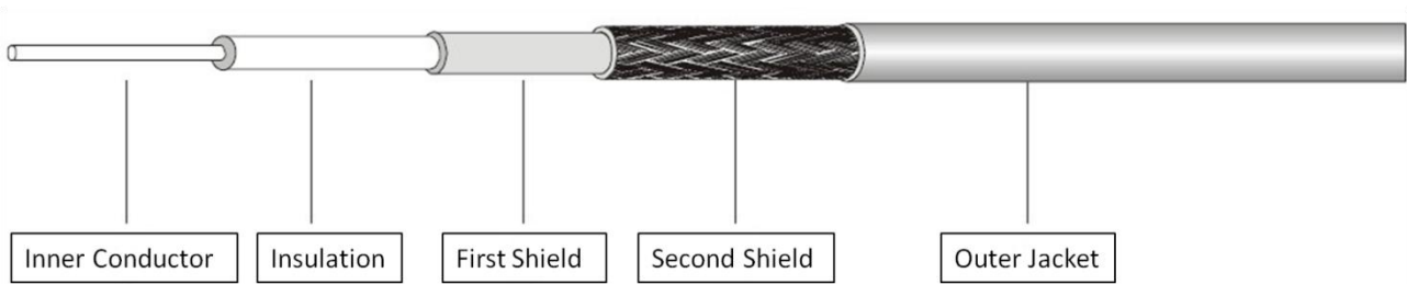
产品截面图 Section Drawing
